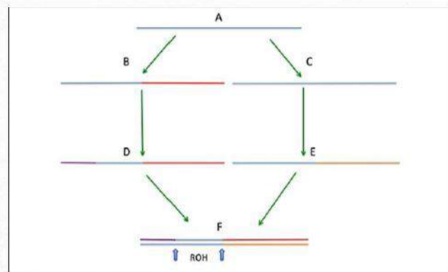
شکل ۱- معیار ROH یکی از روش‌های مورد استفاده برای ارزیابی همخوانی، که نشانگر طول‌های بهم پیوسته ژنوتیپ هموزیگوت انتقال یافته از والدین به فرزندان خود بوده است.
