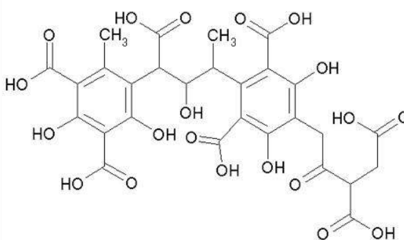
شکل ۱- ساختار مولکولی اسید هیومیک (فالوست، ۱۹۹۸)
